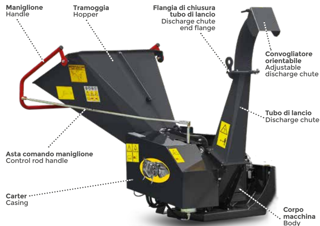
Apertura tramoggia 700x570 mm Hopper 700x570 mm
